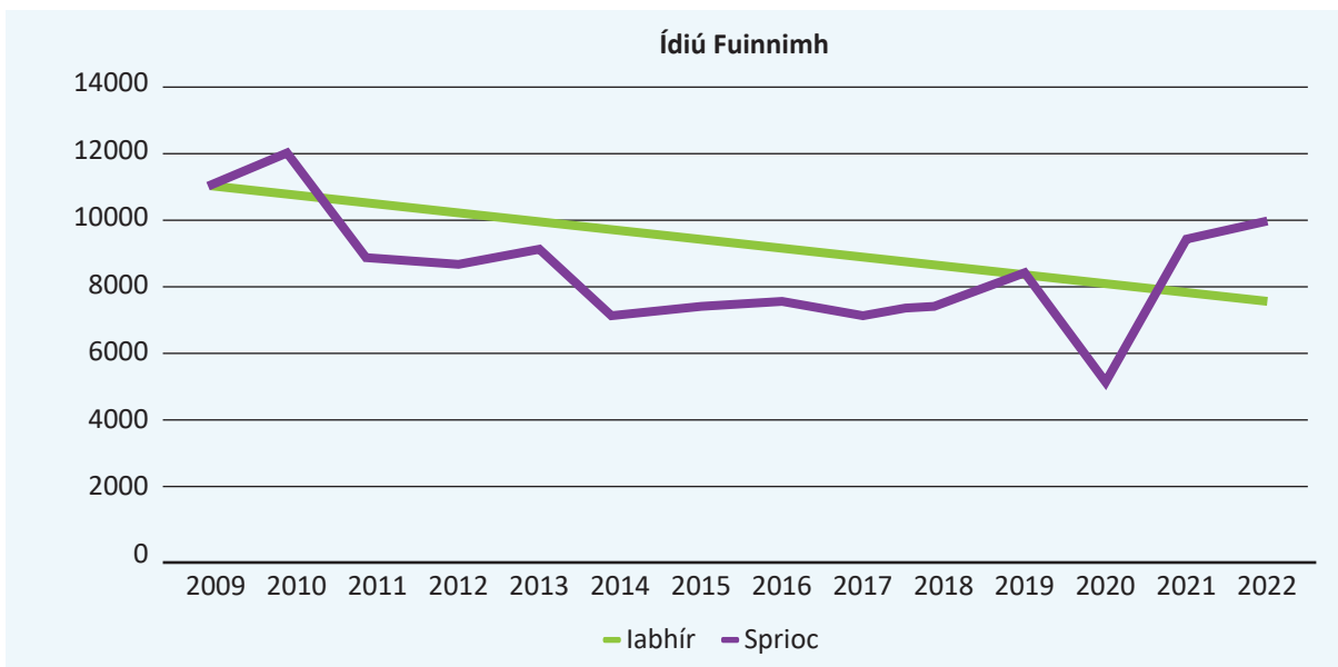
Fíor 7: Táscaire feidhmíochta fuinnimh, Príomhriachtanas Fuinnimh Iomlán in aghaidh gach Fostaí Lánaimseartha, 2009 go 2022.
